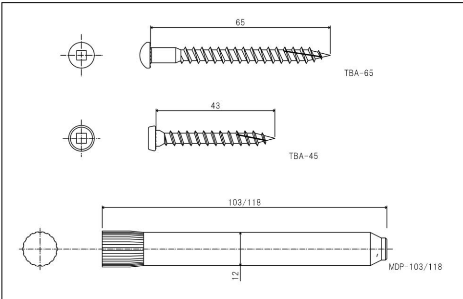
図 5：接合具
