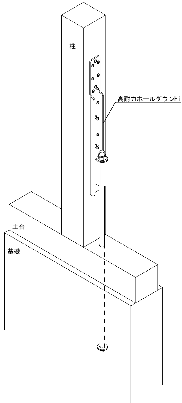
高耐久オメガアンカーボルトM16
