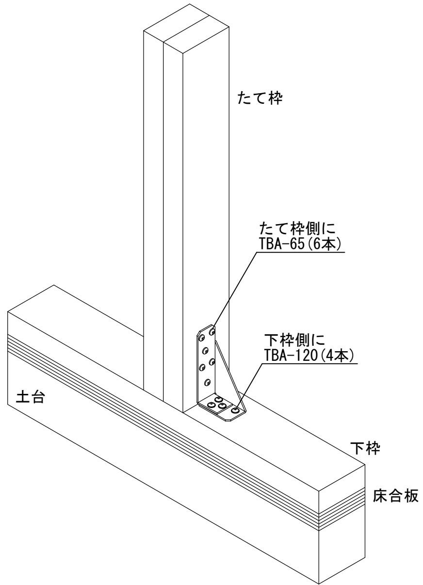
2×4用ホールダウンコーナー〈SW67〉
