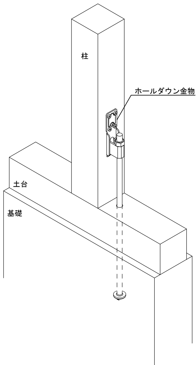
オメガアンカーボルトM16
