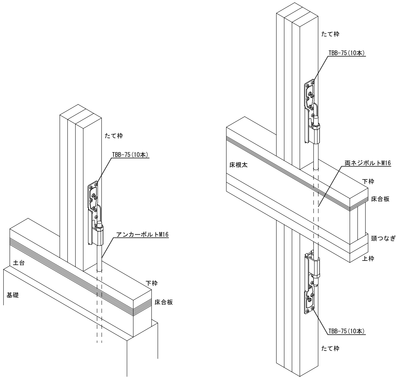
2×4用ビスどめホルダウンHi36
