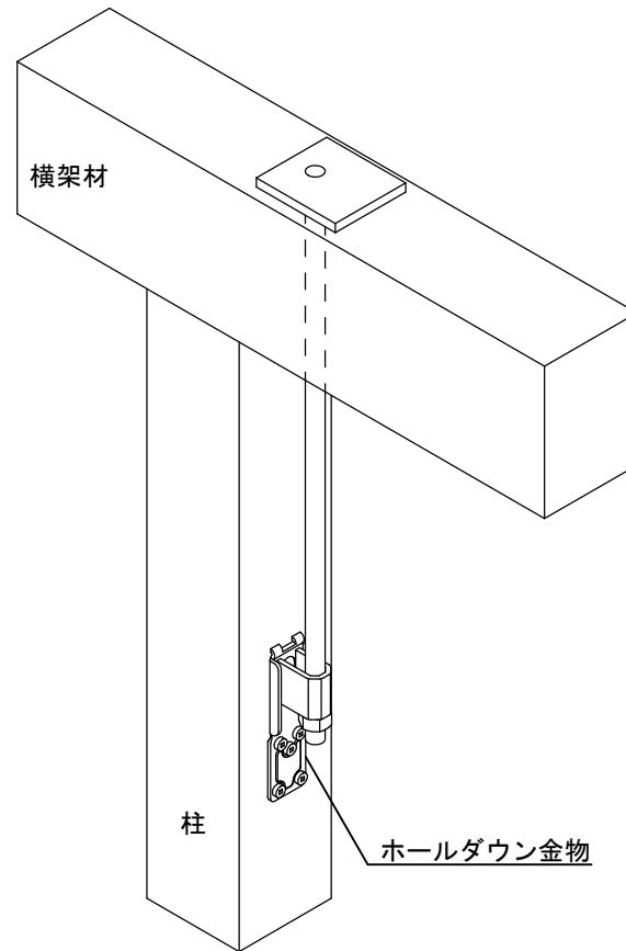
偏心座金付ボルトⅡ
