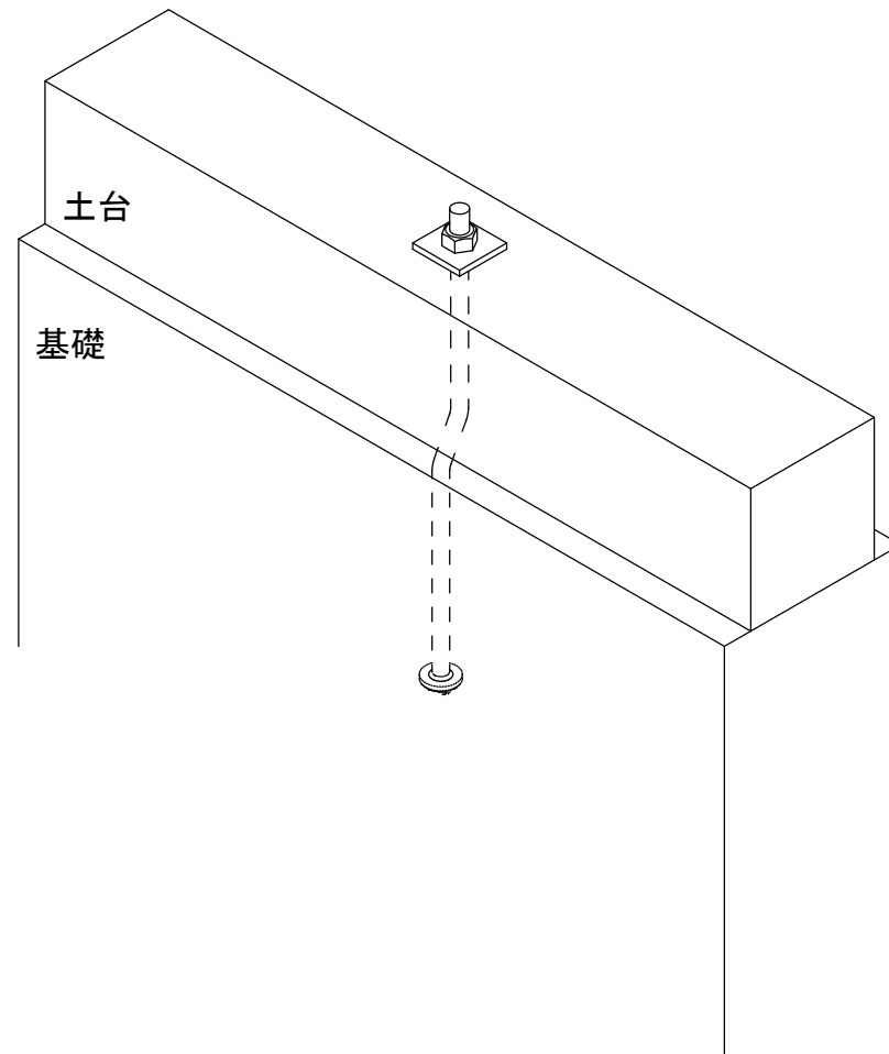
オメガランクアンカーボルトM12
