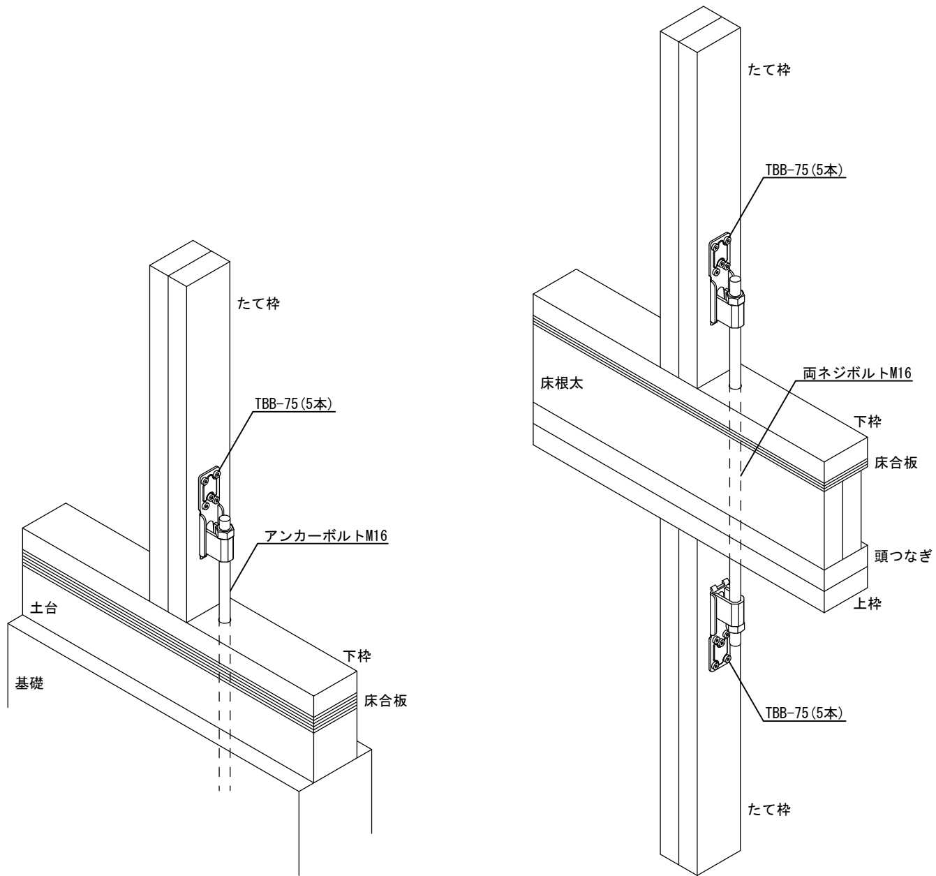
2×4用ビスどめホールダウンHi27
