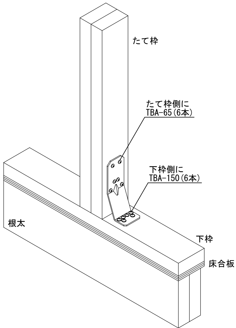
15kN用2×4用オメガコーナー
