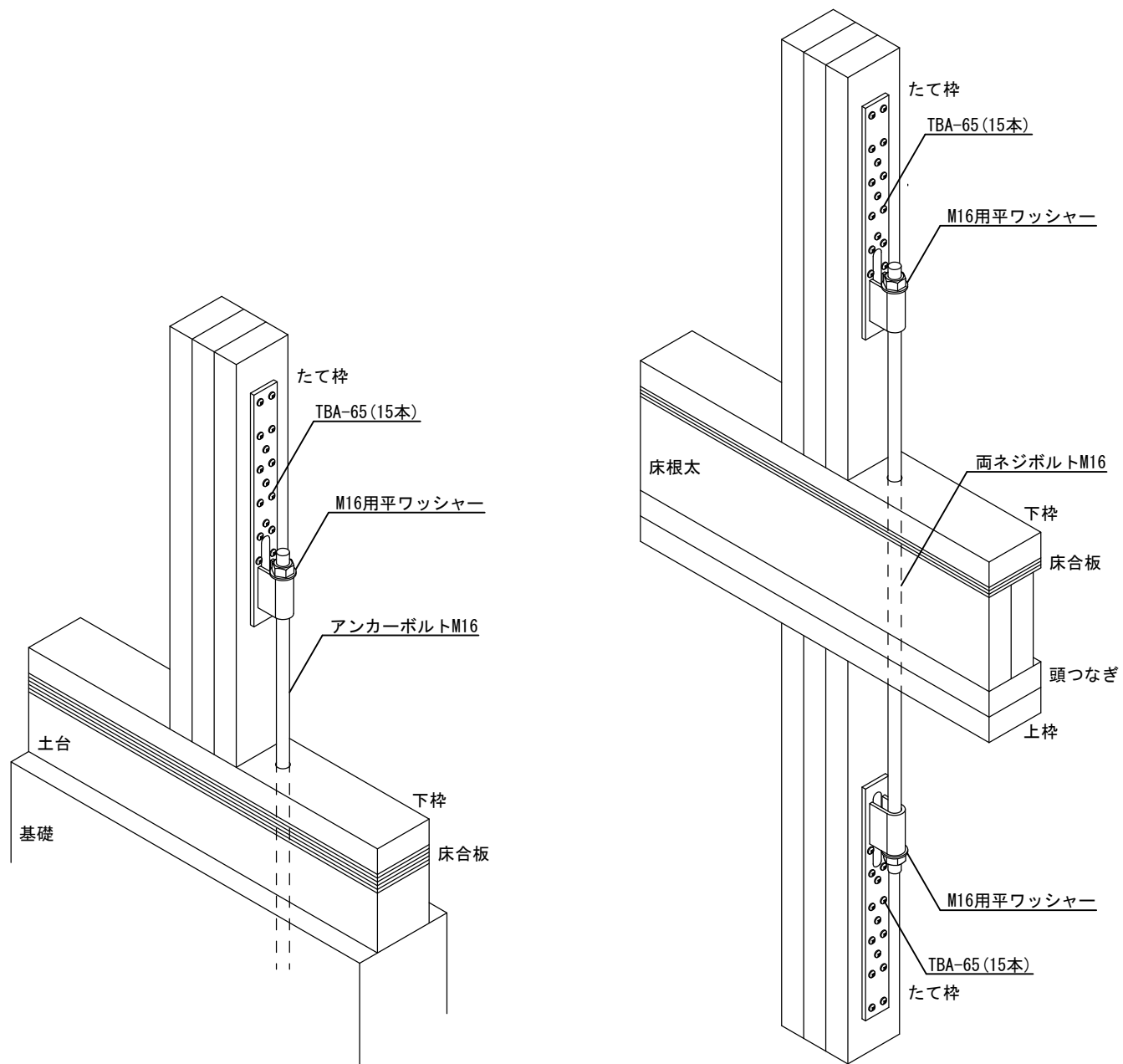
2×4用ビスどめホールダウンU 35kN用
