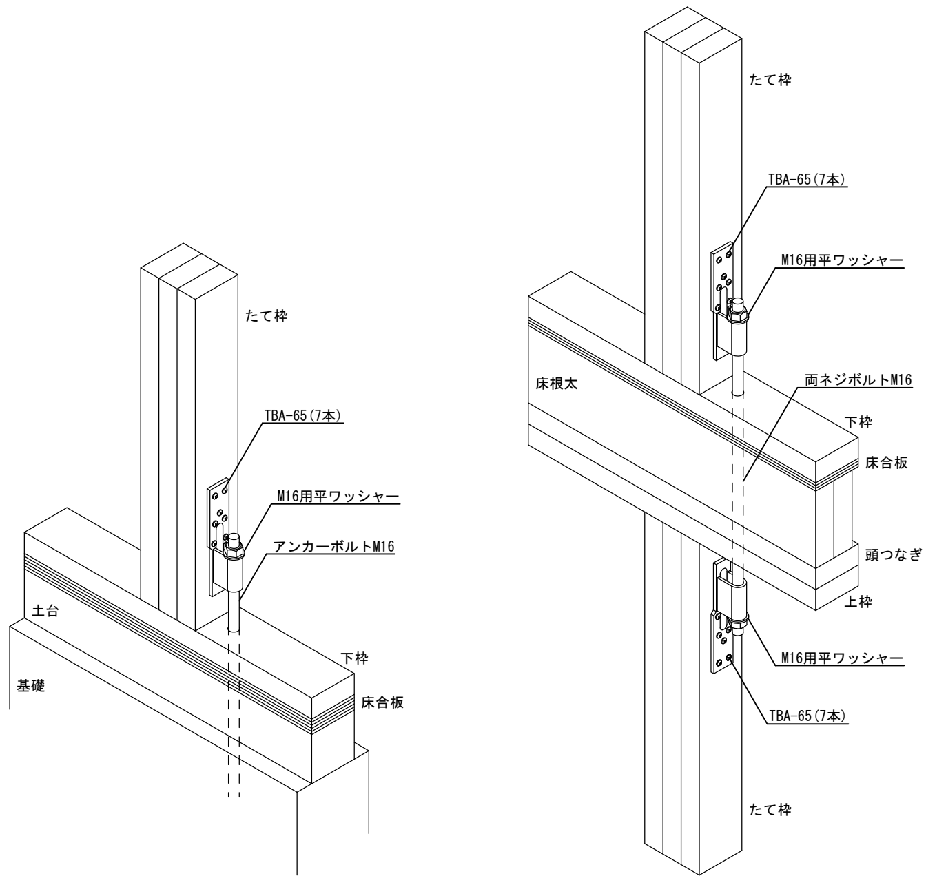
2×4用ビスどめホルダウN 20kN用
