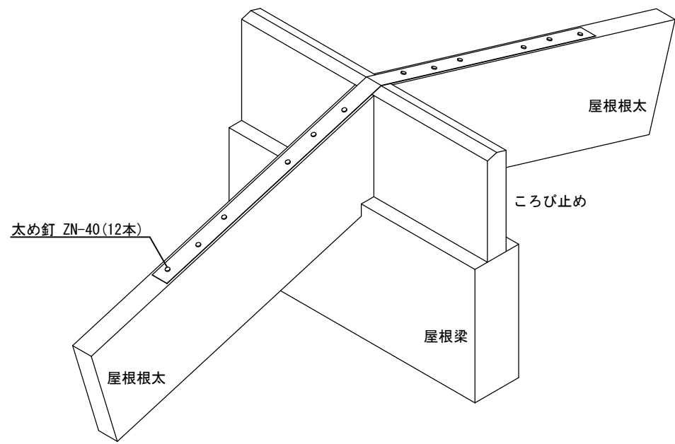
オメガ帯金物 S-90SD
