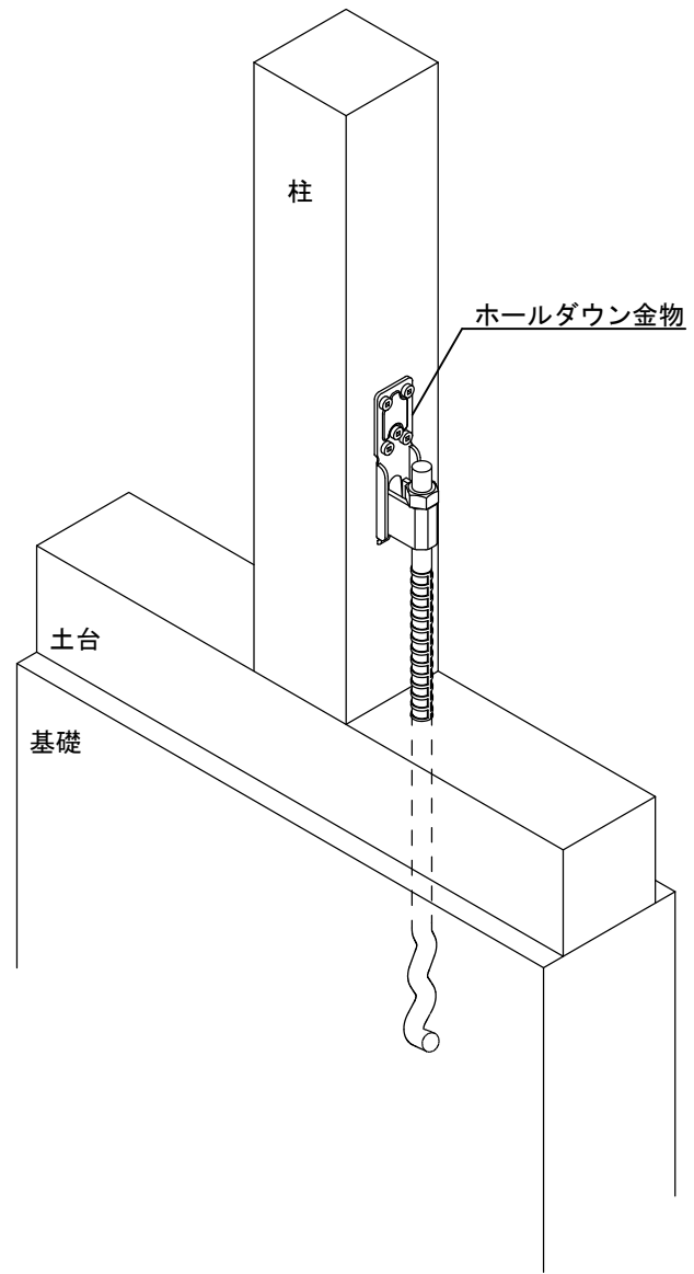
異形Sアンカーボルト
