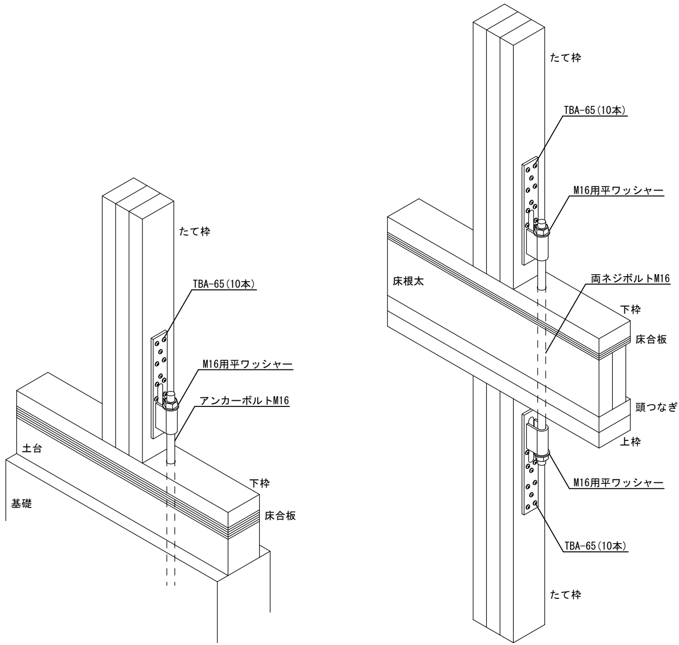
2×4用ビスどめホールダウンU 25kN用
